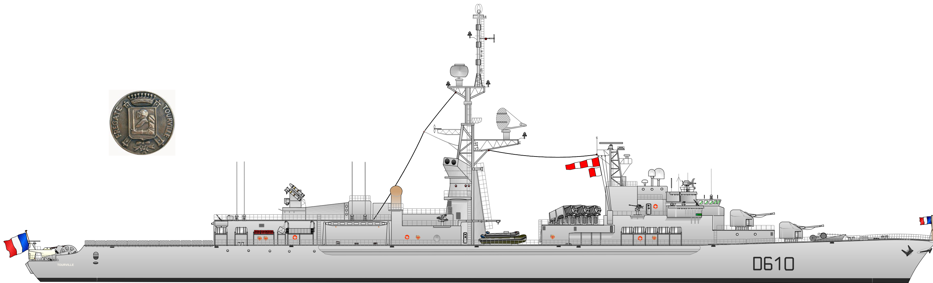
La frégate TOURVILLE appareille de Brest le 4 octobre 2010 pour une mission AGAPANTHE de 5 mois. Le commandant est le C.V. DURTESTE
